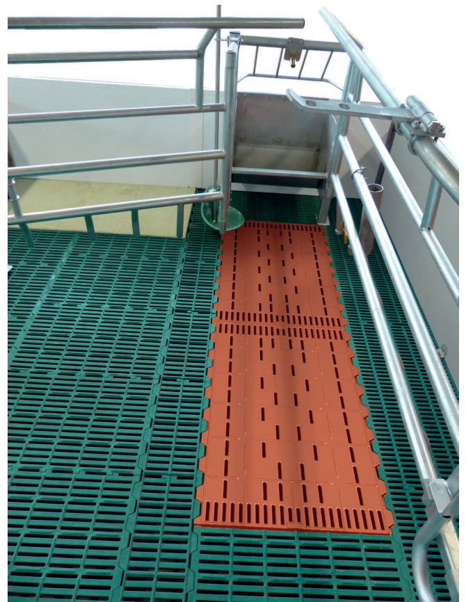
Abb.: Mix-System mit Ferkelnest-Vergrößerungen in Bewegungs-Abferkelbuchten
